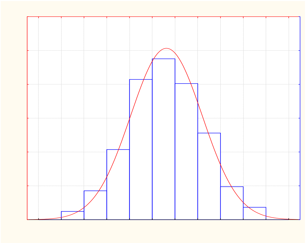
Рисунок Б.7 – Діаграма розподілу вірогідності маси поїздів ділянки Колосівка – Чорноморська
