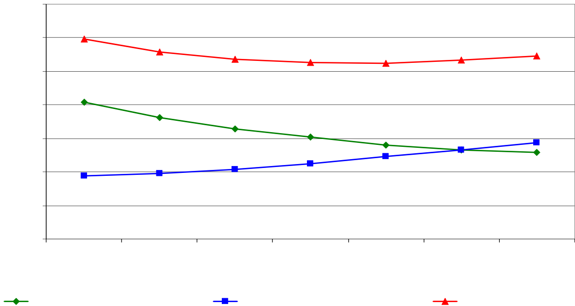
Рисунок 5.2 – Графік змін річних витрат на перевезення розподілювального поїздопотіку по кожній ітерації моделювання на напрямку з паралельними ходами Знам'янка - Одеса
