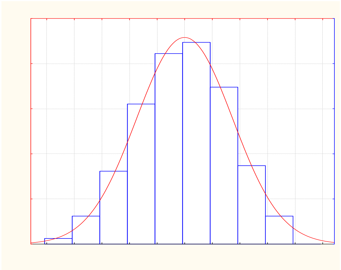
Рисунок Б.10 – Діаграма розподілу вірогідності маси поїздів ділянки Котовськ – Роздільна
