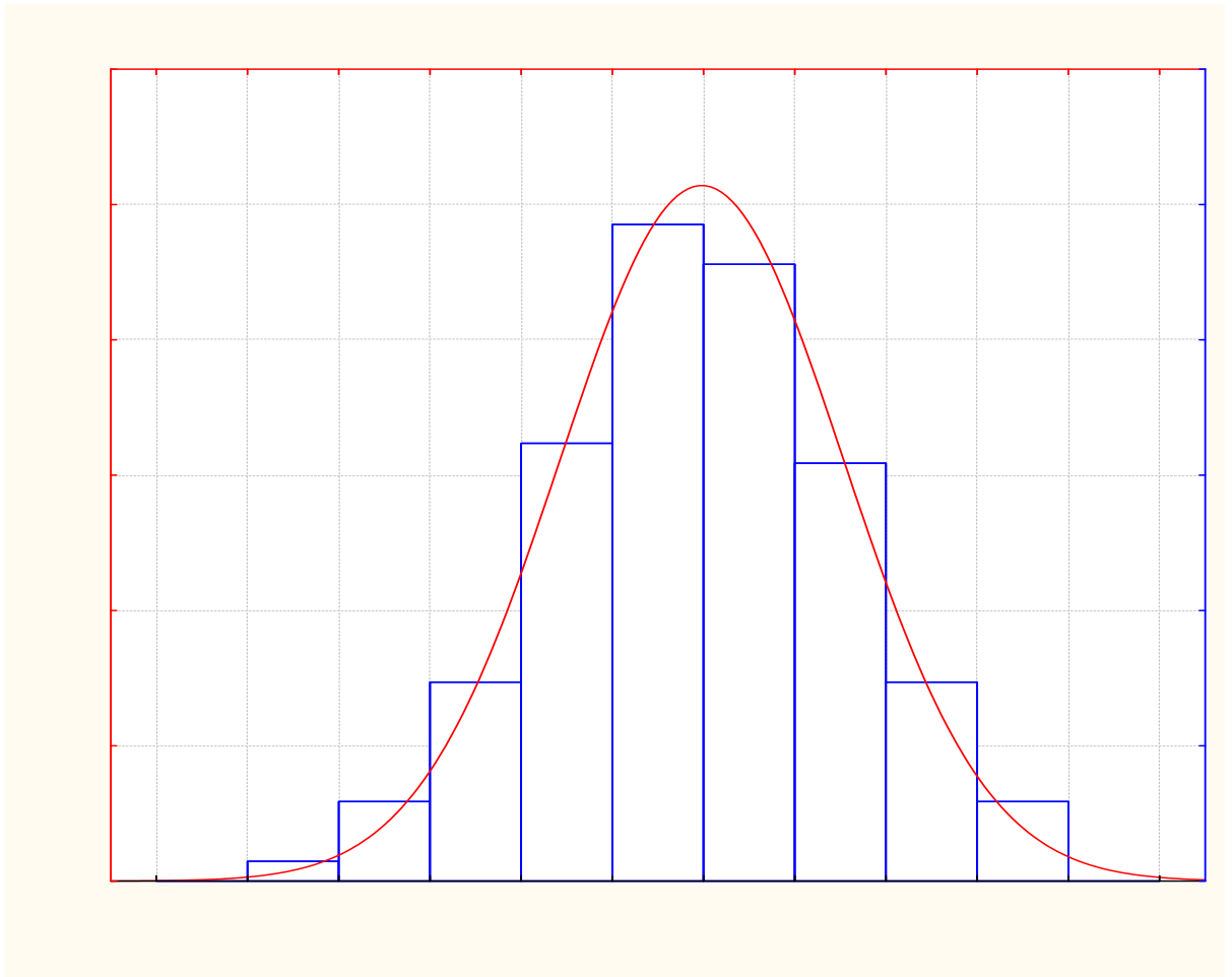
Рисунок Б.12 – Діаграма розподілу вірогідності маси поїздів ділянки Помічна – Котовськ
