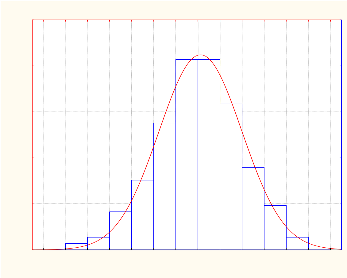
Рисунок Б.4 – Діаграма розподілу вірогідності маси поїздів ділянки Чорноморська – Одеса-Сортувальна
