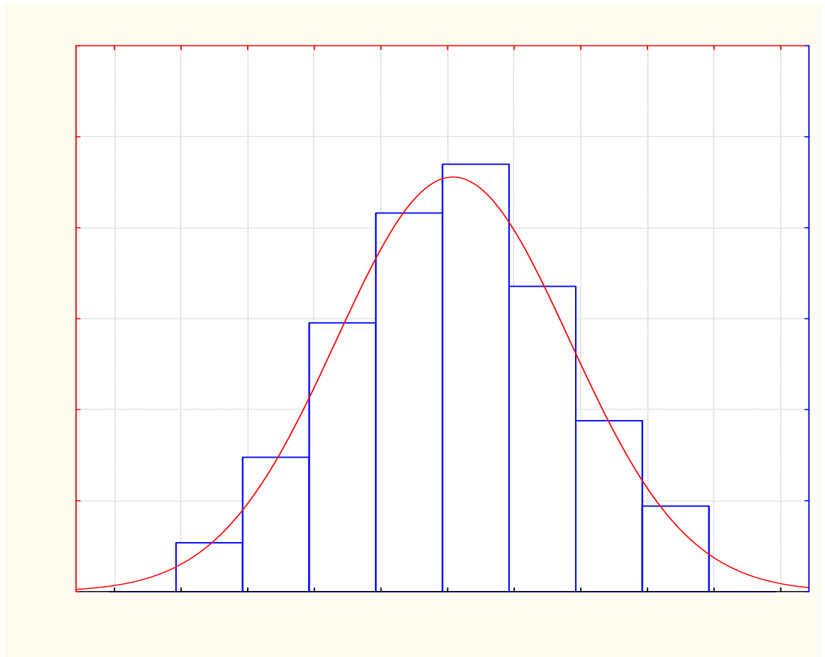
Рисунок Б.9 – Діаграма розподілу вірогідності маси поїздів ділянки Помічна – Котовськ
