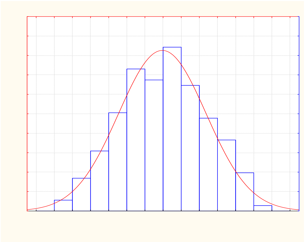
Рисунок Б.11 – Діаграма розподілу вірогідності маси поїздів ділянки Роздільна – Одеса-Сортувальна
