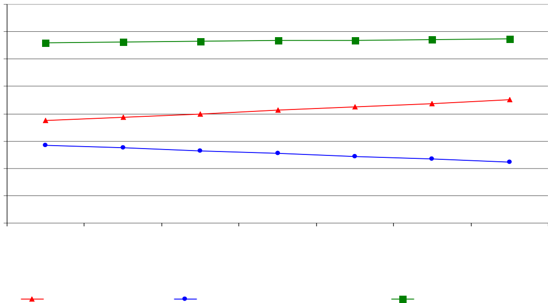
Рисунок 5.4 – Графік моделювання кількості обгонів вантажних поїздів на ділянці основного ходу та загальна кількість зупинок на напрямку з паралельними ходами
