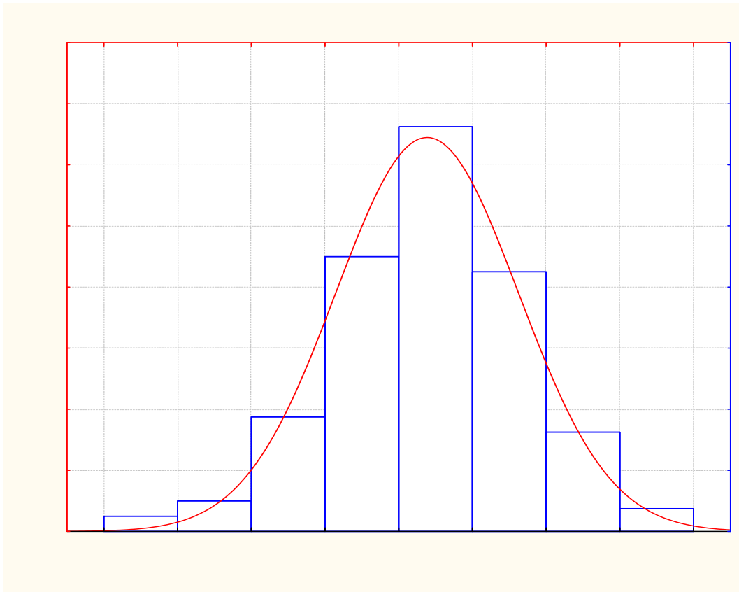
Рисунок Б.2 – Діаграма розподілу вірогідності маси поїздів ділянки Помічна – Колосівка
