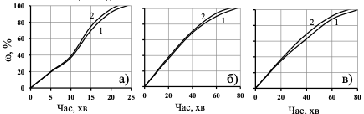
Рис. 10. Кінетика відновлення \text{Fe}_2\text{O}_3 (а), прокатної окалини (б) і магнетитового концентрату (в) графітом у потоці \text{CO} за температури 1173 К, в умовах магнітного поля промислової частоти ( H=24 \text{ кА/м} ): 1-зовні поля; 2-у полі.
