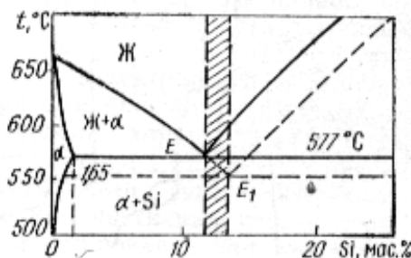
Рисунок 5 – Зміна положення прикордонних ліній діаграми стану системи Al-Si при зміні натрієм. Суцільні лінії – рівноважна діаграма стану [11]
