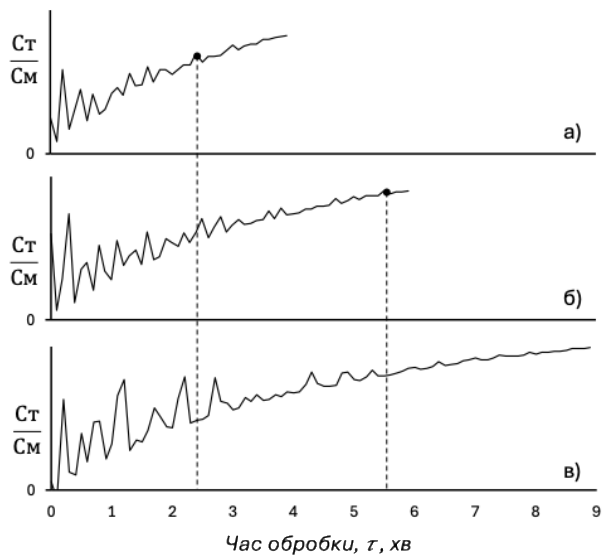
Рис. 5с. З огляду на те, що присадку індикатора проводили в протилежному від датчика боці ковша, у всіх випадках після введення індикатора фіксували збільшення величини \frac{St}{Cm} до моменту, коли значення \frac{St}{Cm} не змінювалося під час подальшого продування.
