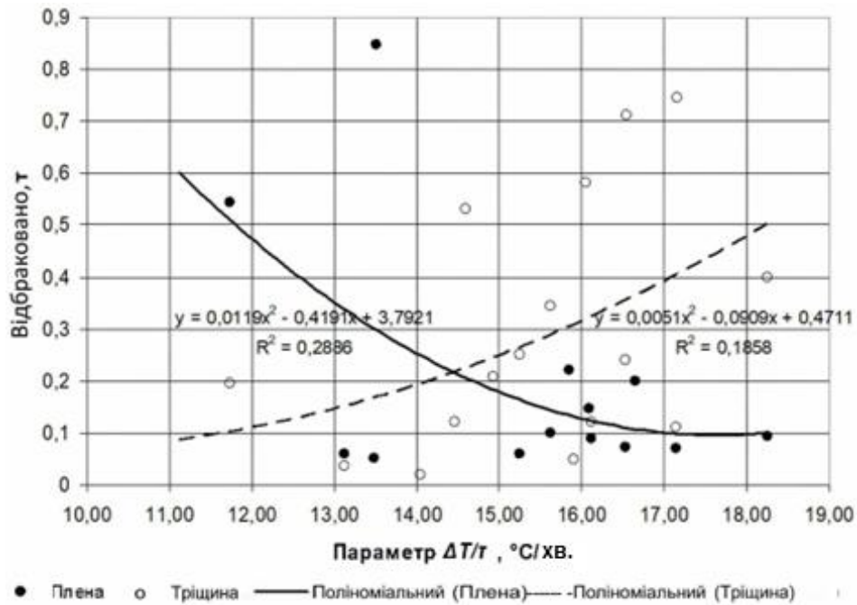
Рисунок 3 – Залежність ураження злитків стали K63 тріщинами та пленами від параметра \Delta T/\tau
