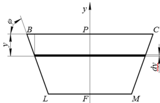
Рисунок 4 – Розрахункова схема визначення площі поперечного перетину частинки
