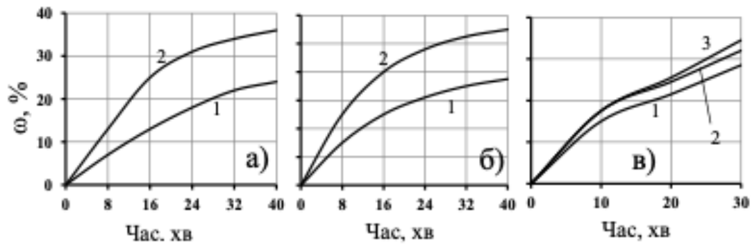
Рис. 11. Вплив високочастотного ЕМП на кінетику відновлення Fe 2 O 3
