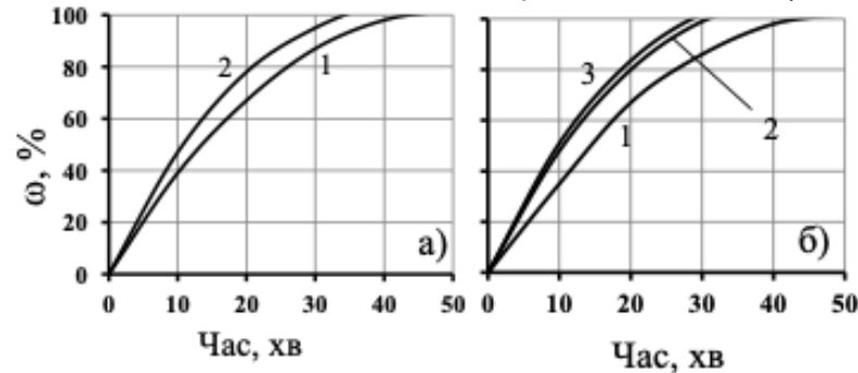
Рис. 13. Вплив ЕМП (f=40 кГц) на кінетику відновлення Fe 2 O 3 сажистим вуглецем у потоці CO за 1073 K, а) зі стабілізацією температури і б) без стабілізації температури: 1-поза полем; 2-під впливом поля (W=50 В); 3-під впливом поля (W=90 В).
