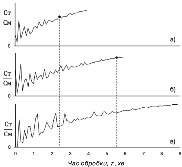
Рис. 5 наведено зміну концентрації індикатора \frac{St}{Cm} у модельовальній рідині під час продування в ковші з різними витратами газу. За відносно великих витрат газу тривалість повного змішування невелика і становить близько 2,5 хв (такий режим можливий при продуванні у ковшах невеликої місткості). Ближчою до звичайної в практиці тривалості продування (5-10 хв.) є динаміка зміни величини \frac{St}{Cm} , наведена на
