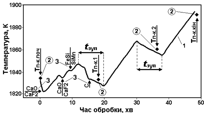
Рис. 2. Зміна температури сталі під час обробки: 1-модельні значення, 2-результати контролю термометрами, 3- введення добавок
