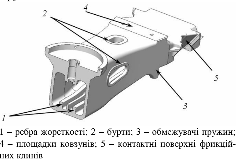
Рисунок 1 – Основні конструктивні елементи бічної рами.
