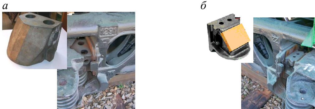
Рисунок 18 – Просторовий (а) та плоский з полімерною накладкою (б) фрикційні клини ресорного підвішування
