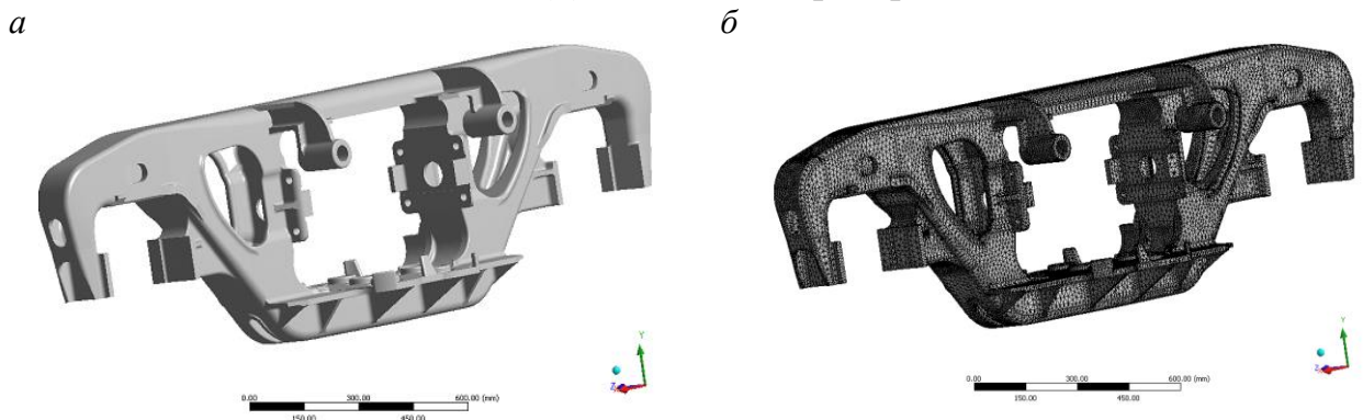
Рисунок 4 – Загальний вид розрахункової ( a ) та скінченно-елементної ( б ) моделей бічної рами
