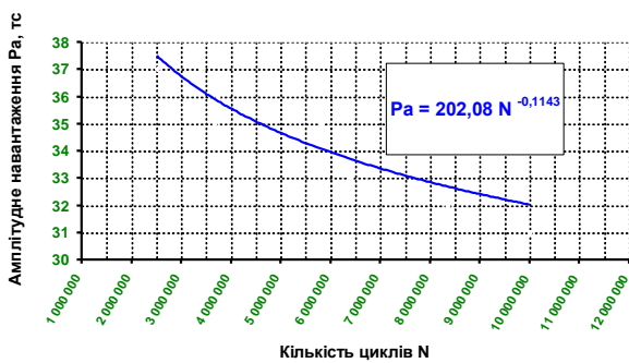
Рисунок 9 – Результати випробувань надресорної балки (а), бічної рами (б) на втому
