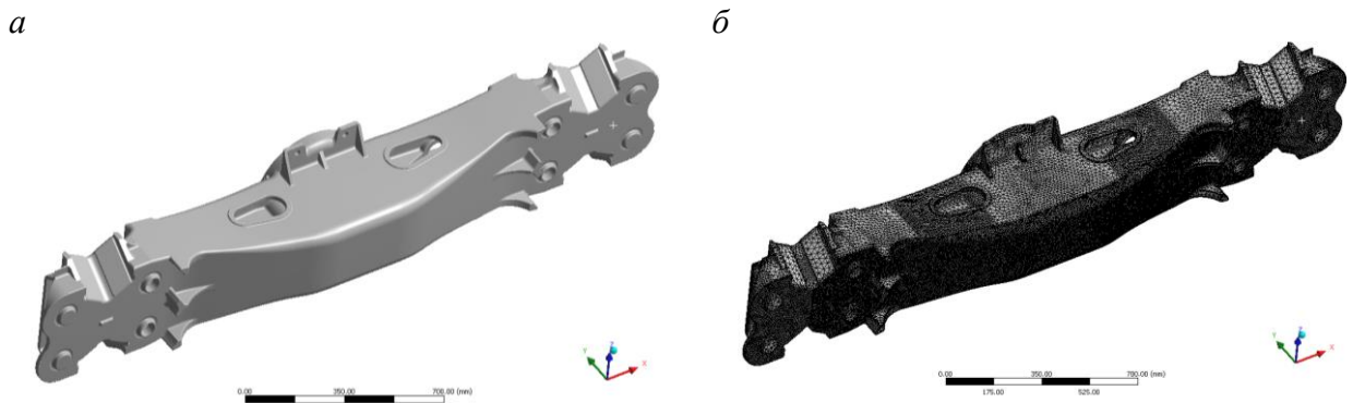
Рисунок 3 – Загальний вигляд розрахункової ( a ) та скінченно-елементної ( б ) моделей надресорної балки
