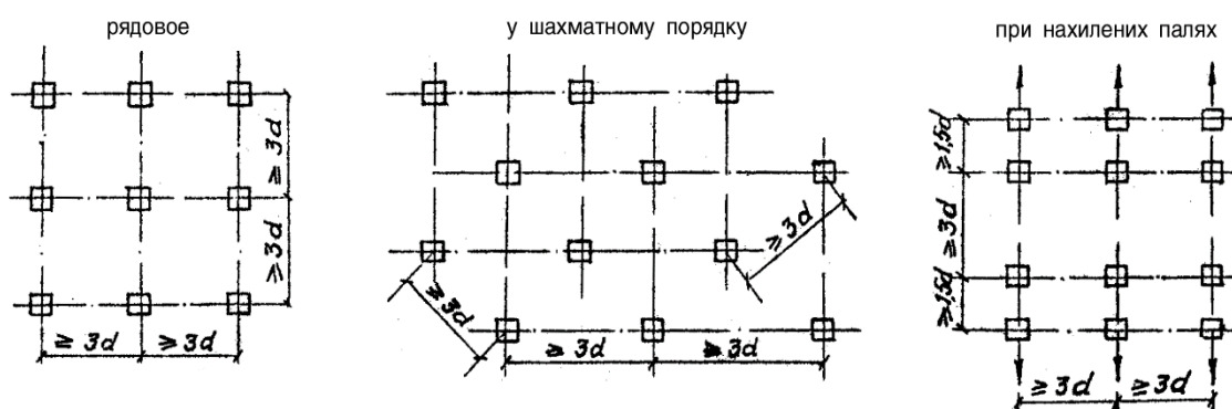
Рис. 10.3. Розміщення паль у площині підшви ростверку
