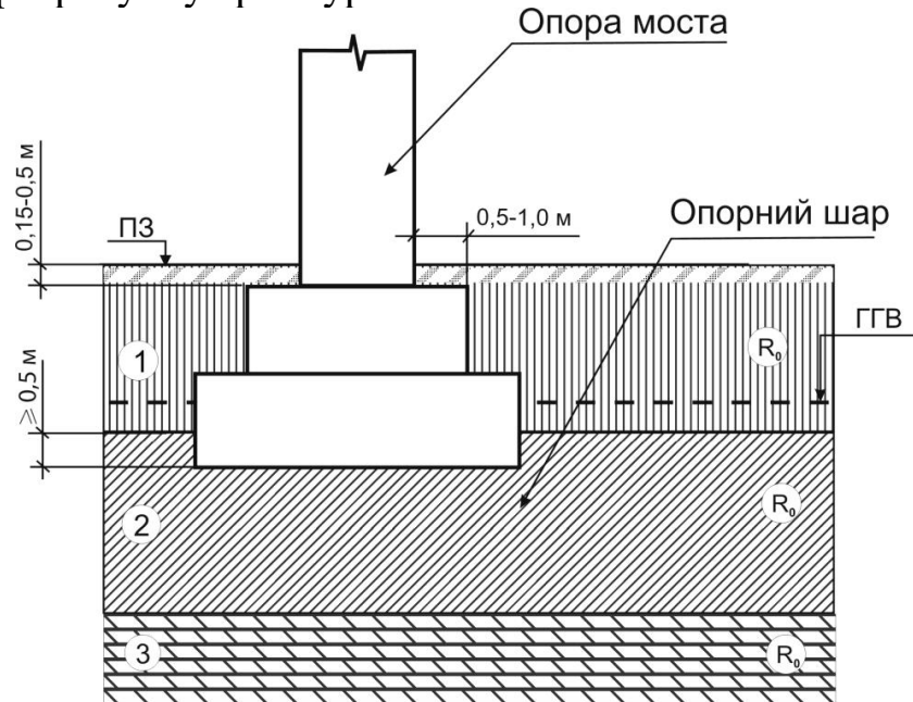
Рис. 3.2. Масивний фундамент мілкового закладання на суходолі
