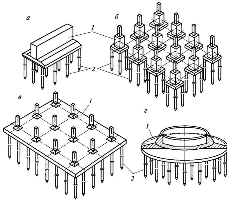
Рис. 1.9. Типи фундаментів глибокого закладення (пальових) для промислового та цивільного будівництва: а – стрічковий ростверк; б – стовчатий ростверк; в, г – плитно-пальовий; 1 – фундамент; 2 – забивні палі
