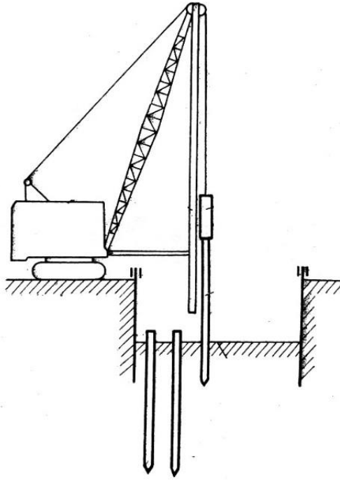
Рис. 14.1. Забивка паль з поверхні котловану
