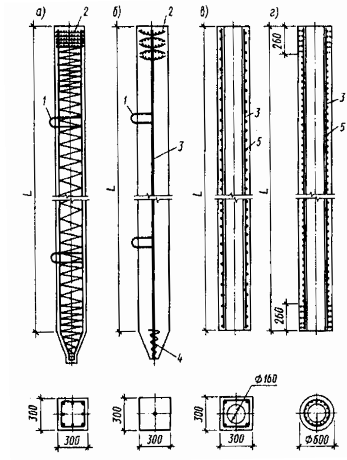
Рис. 9.3. Види армування паль:
