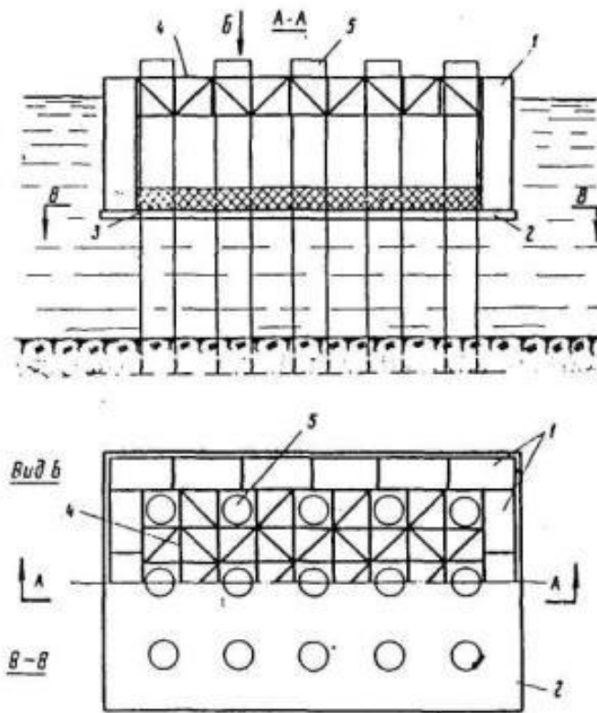
Рис. 16.2. Огороження з інвентарних понтонів типу КС
