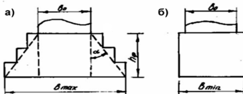
Рис. 3.1. Фундаменти: а – з розширеною підшвою; б – без розширення.
