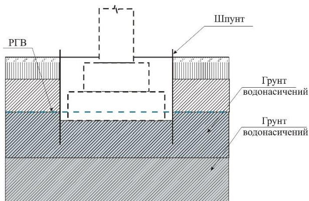
Рис. 6.8. Схема котловану з рівнем ґрунтових вод вище дна котловану та забитим шпунтом
