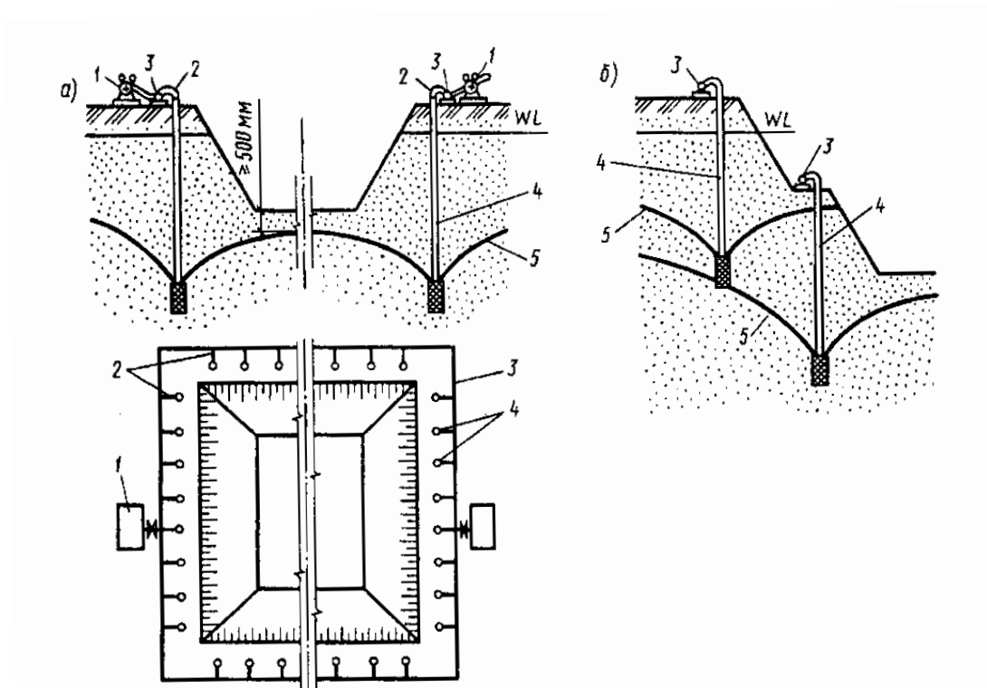
Рис. 8.1. Схеми глибинного водозниження:
