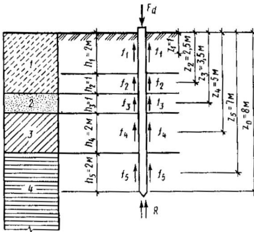
Рис. 10.2. Схема розрахунку несучої здатності паль по ґрунту
