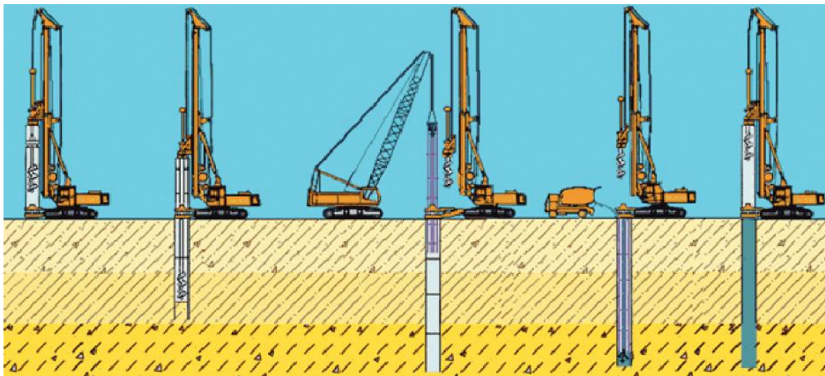
Рис. 13.6. Виготовлення буронабивних палів
