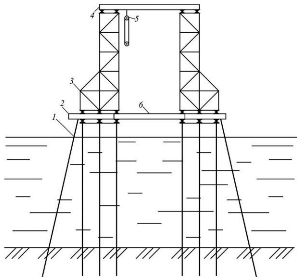
Рис. 15.5. Стационарні підмостки
