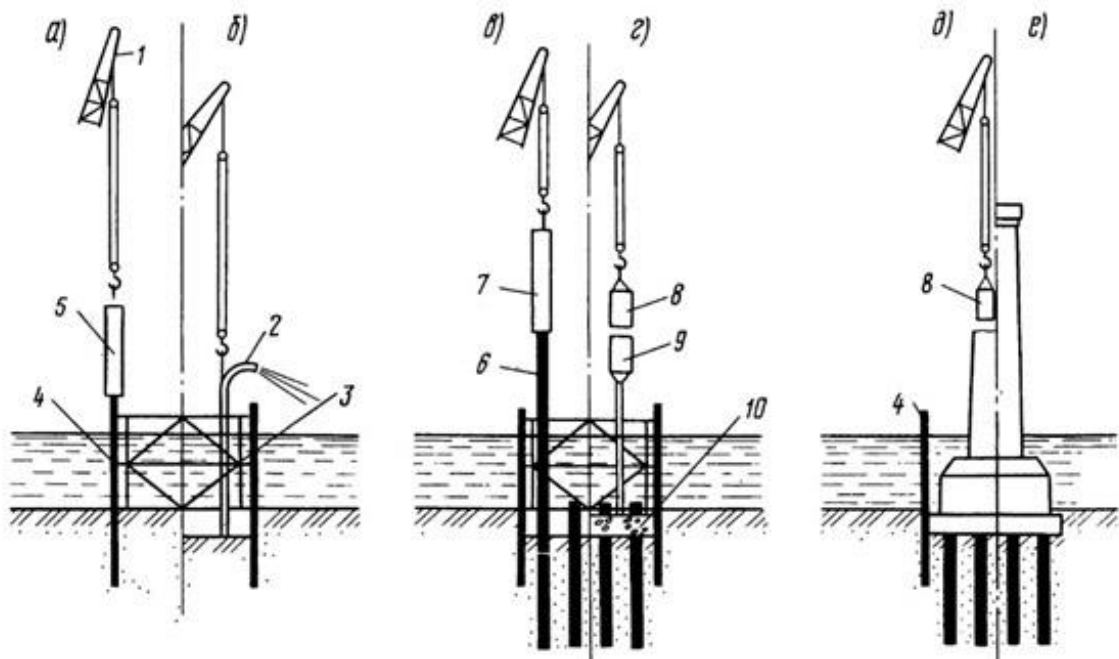
Рис. 15.7. Послідовність будівництва пальового фундаменту із заглибленим у ґрунт ростверком:
