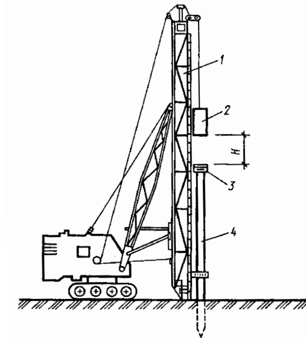
Рис. 13.1. Копер для забивання палі
