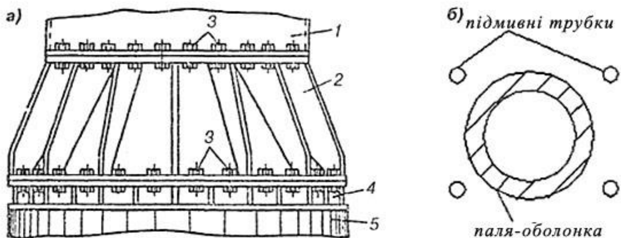
Рис. 16.8. Вібростіп при зануренні палі-оболонки
