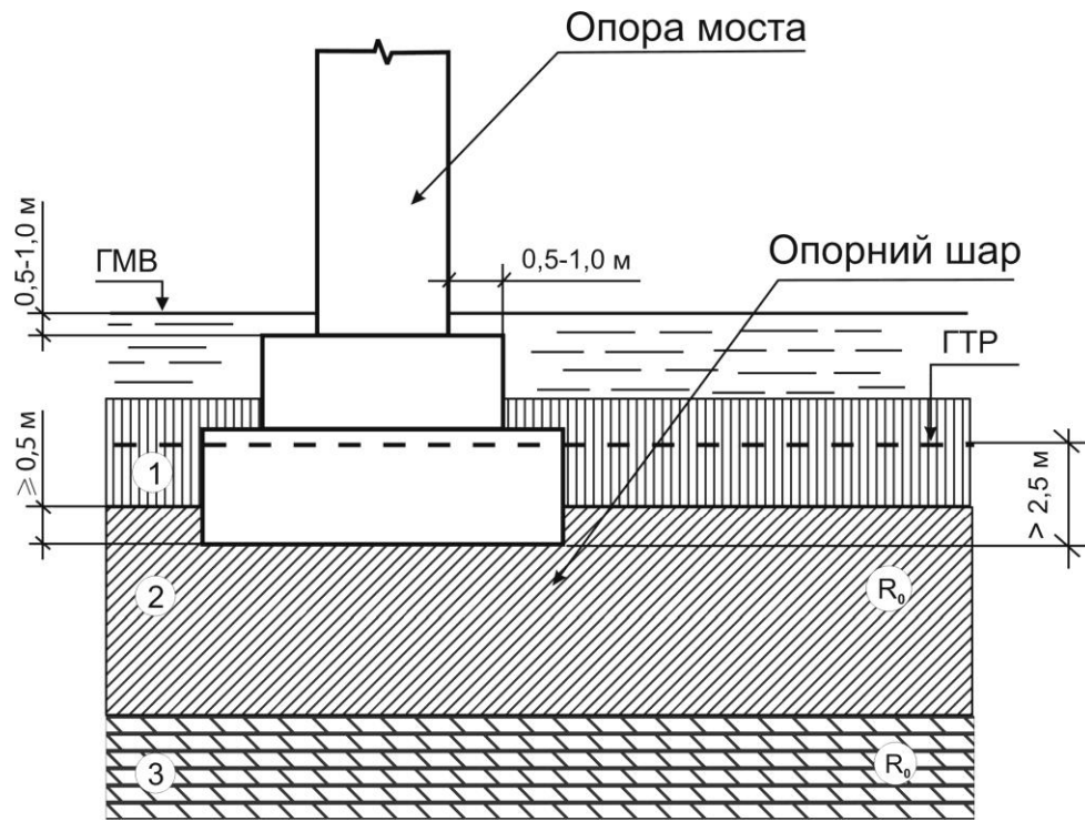
Рис. 4.2. Конструкція фундаменту мілкового закладення на водотоці
