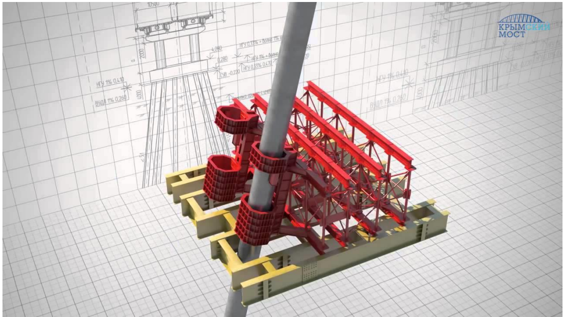
Рис. 16.9. Кондуктор для занурення паль-оболонки
