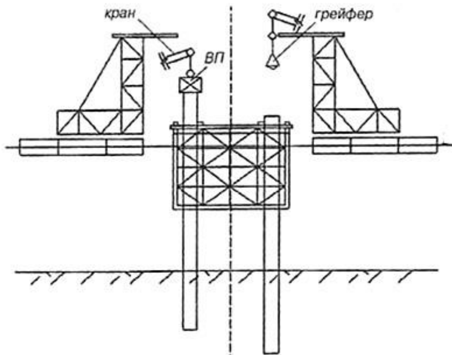
Рис. 16.7. Занурення паль-оболонки з наросуванням секцій і розробкою ґрунту із внутрішніх порожнин оболонки
