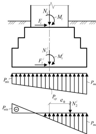
Рис. 4.3. Епюри напружень під підшвою фундаменту
