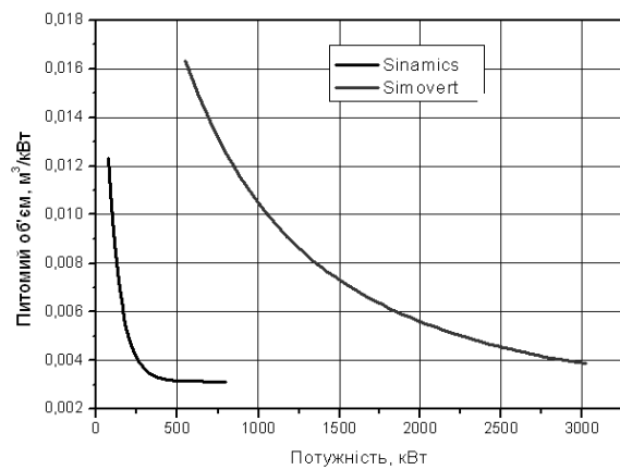
Рис. 7. Залежність питомого об'єму перетворювачів серії Sinamics (380...690 В) та Simovert (2,3...4,16 кВ) фірми Siemens від потужності перетворювачів
