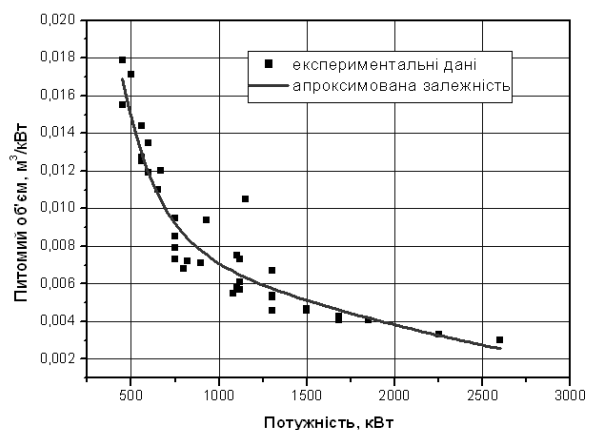
Рис. 12. Залежність питомого об'єму високовольтних перетворювачів серії PowerFlex фірми Rockwell Automation (елементна база – SGCT, з примусовим повітряним охолодженням)
