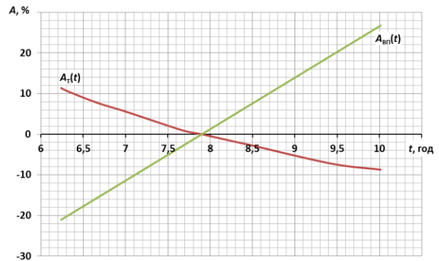
Рис. 3. Залежності відносних відхилень витрат електроенергії від часу руху на ділянці «Знам'янка-Сортувальна – Одеса-Сортувальна»
