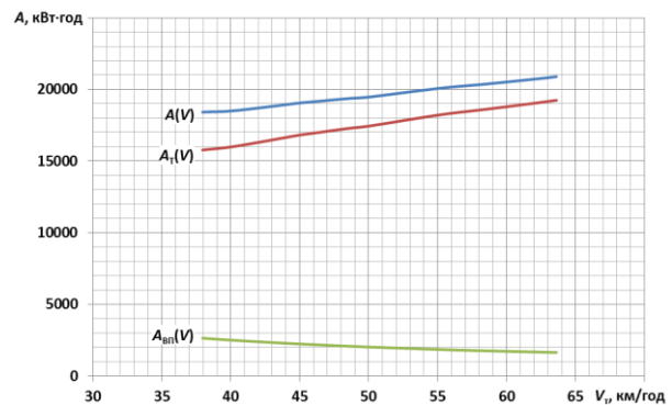
Рис. 4. Залежності витрат електроенергії від технічної швидкості на ділянці «Знам'янка-Сортувальна – Одеса-Сортувальна»
