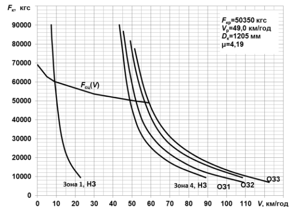
Рис. 1. Тягова характеристика електровоза 2ЭС5К
