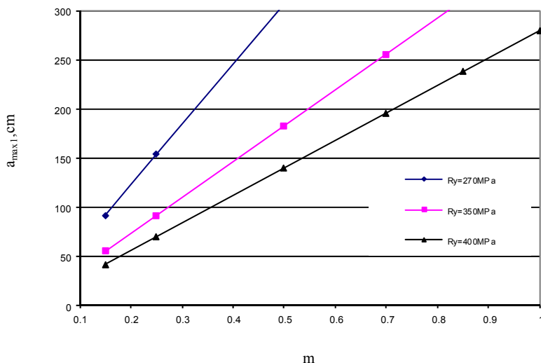
Fig. 2. Relation entre la distance maximale admissible des noeuds de jonction des éléments avec le parement et les caractéristiques géométriques des profils
