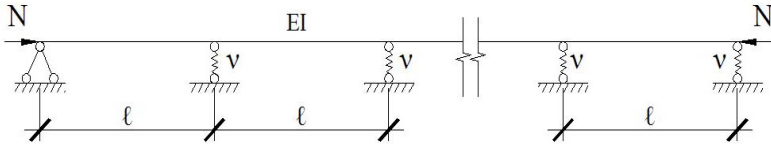
Fig. 3. Schéma de calcul du profil comprimé aux supports élastiques.
