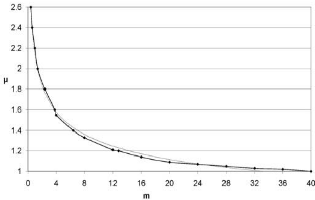
Fig. 4. Relation entre le coefficient de la longueur de calcul \mu et du coefficient de la rigidité m pour le profil comprimé continu sur les supports élastiques [4]
