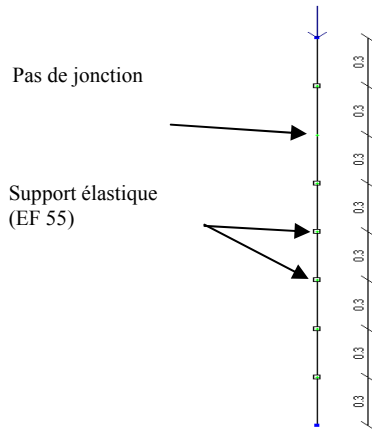
Fig. 5. Schéma de calcul du profil pour la définition des coefficients de longueur de calcul
