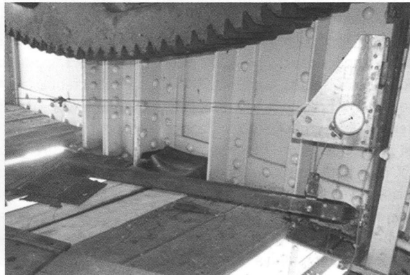
Прилад, розроблений співробітниками лабораторії для вимірювання рівномірності натягу канатів вертикально-підйомної прогонової будови
