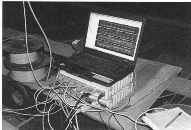
Вимірювальний комплекс із підсилювачем «Spider 8» для реєстрації прогинів та напружень в елементах прогонових будов мостів
