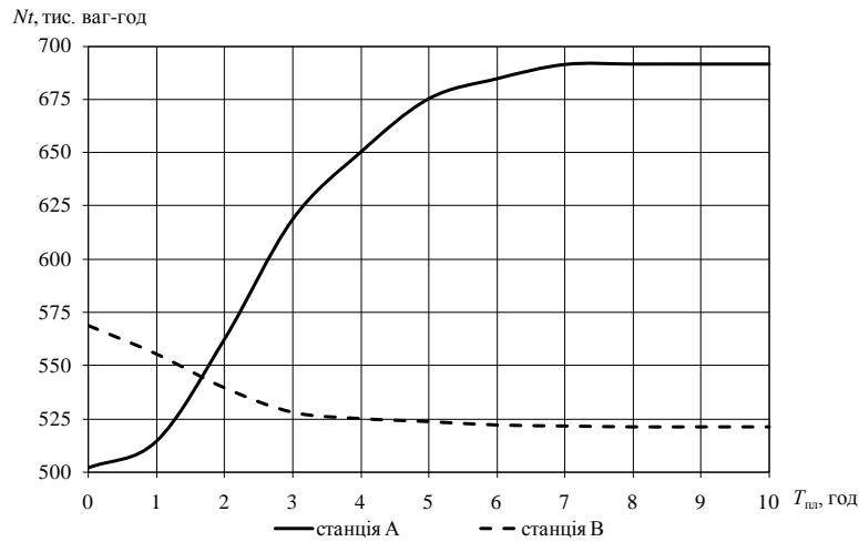
Рис.3. Залежність загальних вагоно-годин простою вагонів призначень В та С від періоду планування
