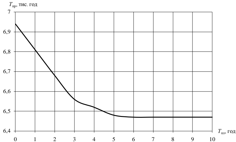
Рис.5. Залежність простою поїзних локомотивів на станції В від періоду планування
