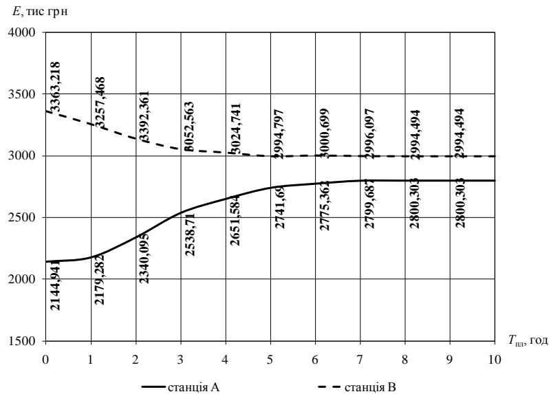
Рис.6. Залежність експлуатаційних витрат на організацію вагонопотоків від періоду планування
