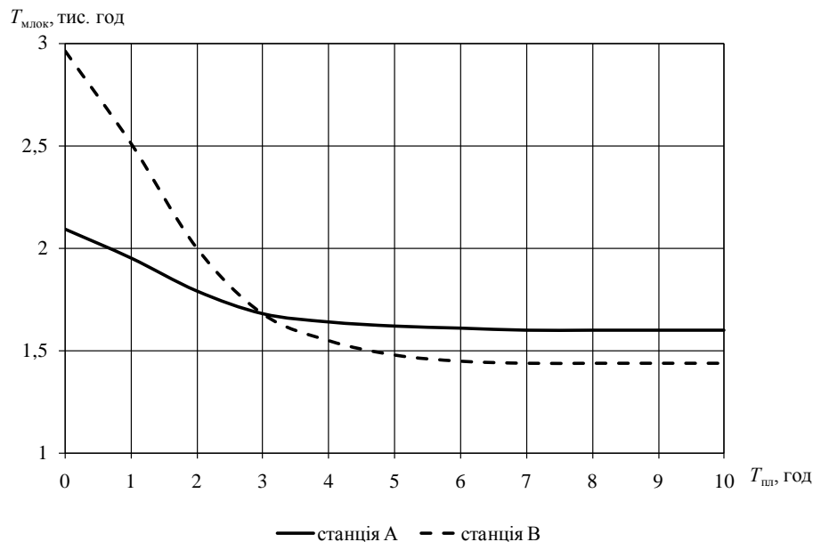
Рис.4. Залежність обсягу маневрової роботи на станціях залізничного напрямку від періоду планування
