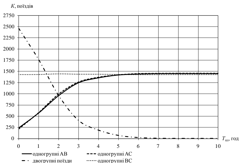
Рис.2. Залежність кількості сформованих одногрупних та двогрупних поїздів від періоду планування
