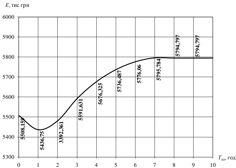
Рис.7. Залежність експлуатаційних витрат по організації вагонопотоків на напрямку А–В–С від періоду планування
