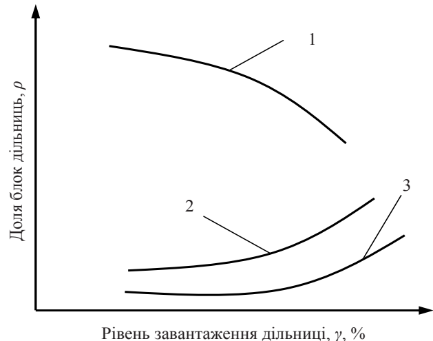
Рис. 5. Залежність долі ( \rho ) блок-дільниці, яку поїзди проходять на зелений (1), жовтий (2) та червоний (3) сигнали світлофорів від рівня заповнення дільниці поїздами ( \gamma )
