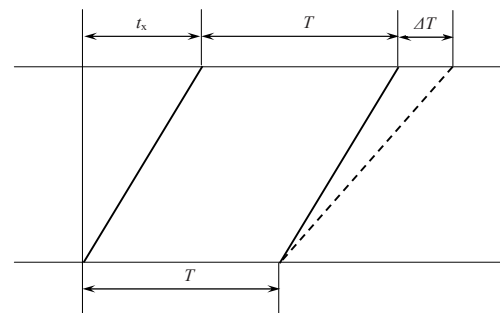
Рис. 6. Фрагмент графіка руху поїздів
