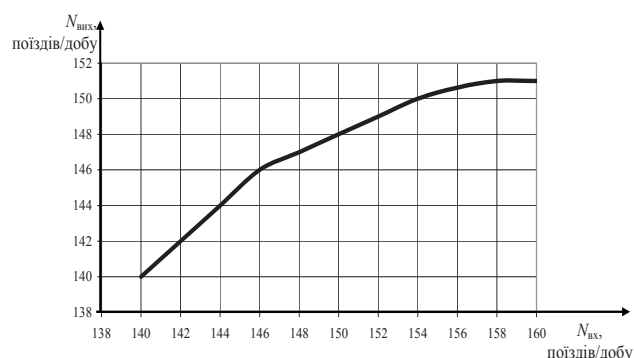
Рис. 7. Графік залежності вихідного і вхідного потоків від густини поїздів на дільниці
