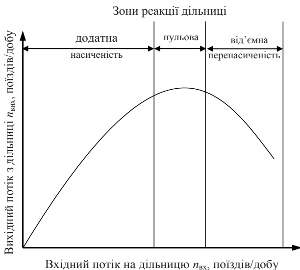
Рис. 4. Реакція дільниці на змінення інтенсивності потоку поїздів
