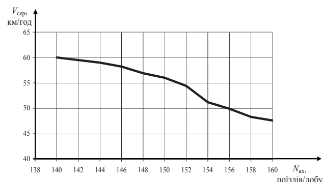
Рис. 8. Графік залежності вхідного потоку N_{\text{вх}} і швидкості руху V
