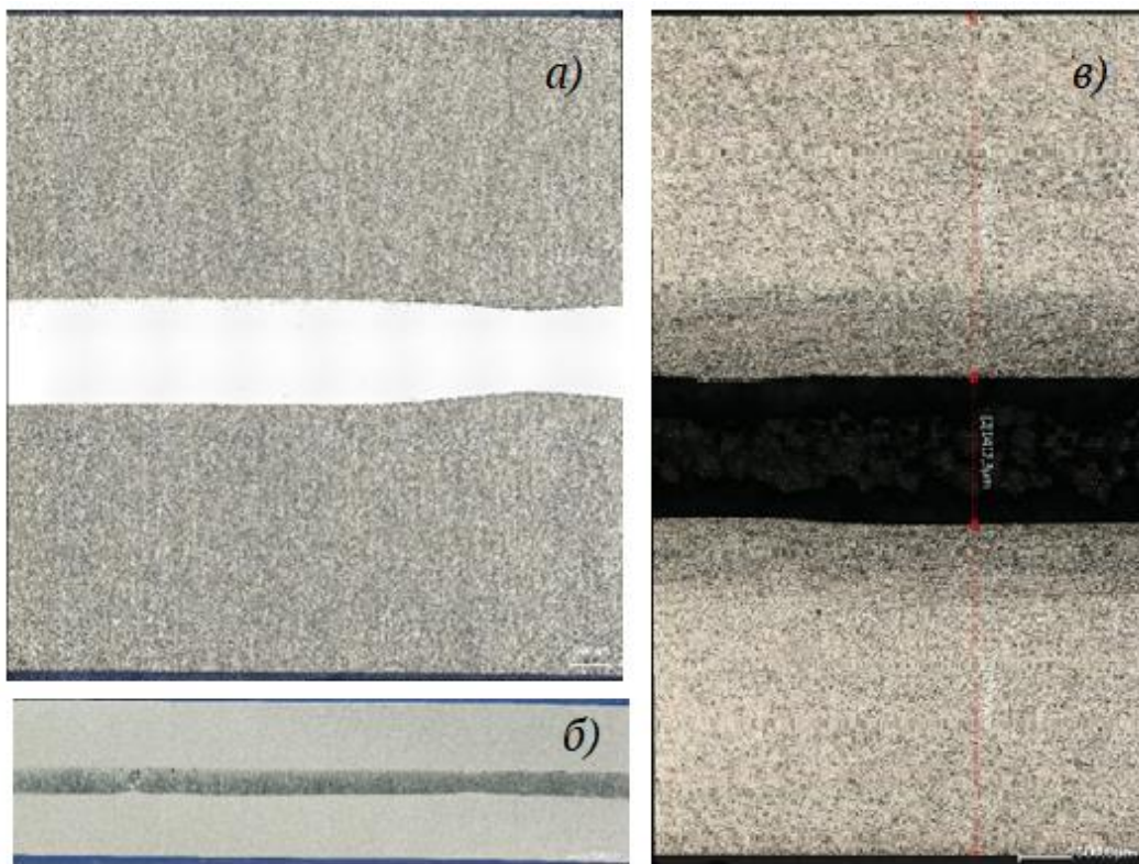
Рисунок 3 – Поперечний переріз тришарової штаби: a – двадцятикратне збільшення; б - десятикратне збільшення; в – десятикратне збільшення у темному полі мікроскопу з розмірами шарів
