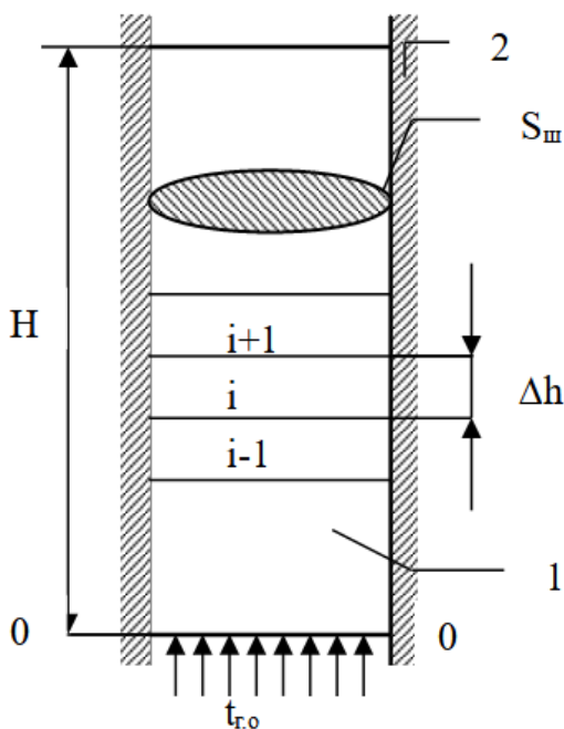
Рисунок — Схема розрахунку: 1 - шар матеріалу, 2 - шахта (камера).
