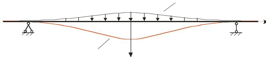
Рисунок 2.10 – Розрахункова схема прогину балки при обпиранні на опори
