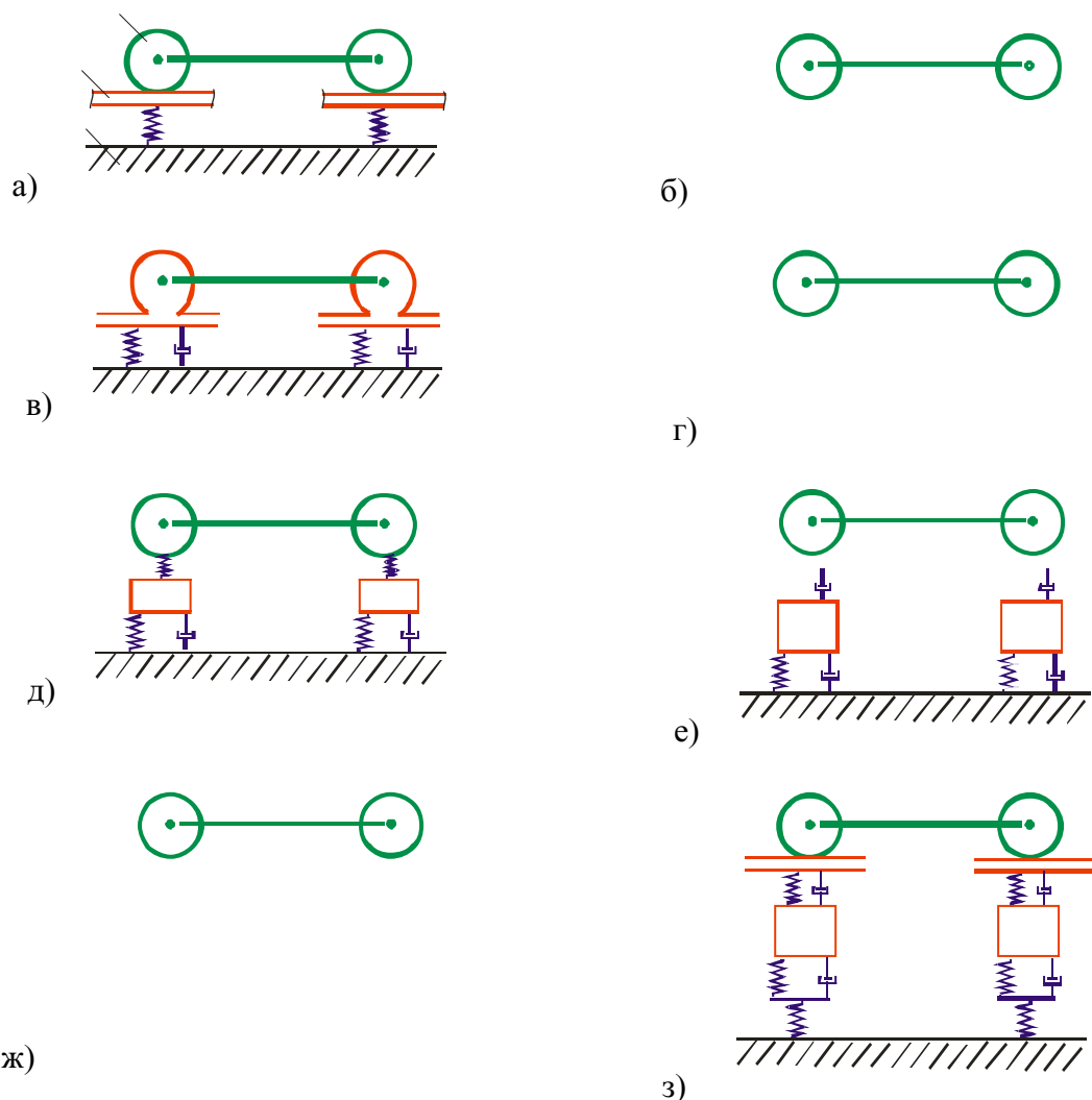
Рисунок 5.11 – Варіанти введення залізничної колії в модель на основі системи рівнянь за принципом Лагранжа-д'Аламбера: 1 – колесо; 2 – рейка; 3 – підрейкова основа; 4 – умовний об'єкт з масою колії, приведеною до одного колеса; 5
