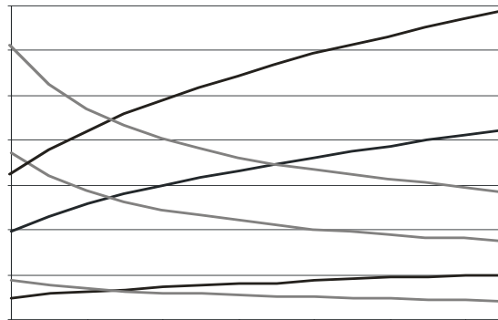
Рисунок 2.4 – Залежність середньоквадратичного відхилення сили від проходження колеса по рейковій нерівності відносно модуля пружності підрейкової основи: 1 – за формулою (2.20); 2 – за формулою (2.24)
