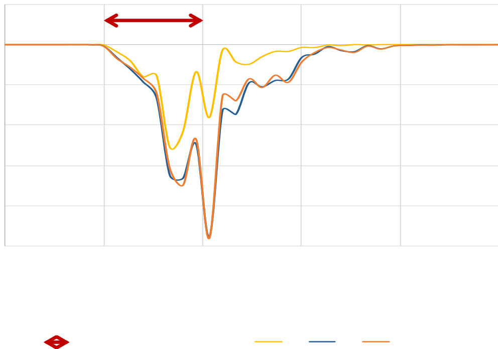
Рисунок 6.5 – Моделювання розвитку нерівності колії для різних варіантів стану ділянки: 1 – вихідна нерівність; 2 – нерівність, утворена з врахуванням впливу первинної зони нерівнопружності; 3 – нерівність, утворена з вихідної з умов поновлення рівнопружності ділянки
