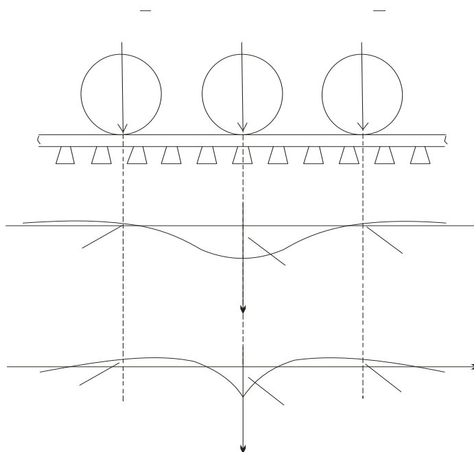
Рисунок 2.7 – Навантаження від трьохвісного візка [20]: а – схема трьохвісного візка; б – лінія впливу коефіцієнта \eta(x) ; в – лінія впливу коефіцієнта \mu(x)
