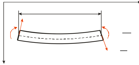
Рисунок 3.23 – Розрахункова схема вигину елементу балки
