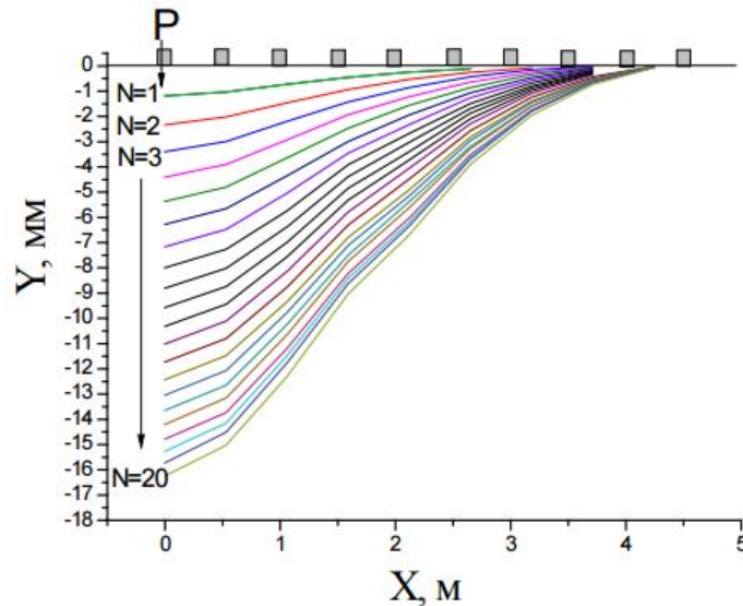
Рисунок 6.1 – Результати розрахунків ітераційного FEM моделювання осадки колії [165]: — зовнішнє навантаження; — осадка; — відстань від точки дії сили; — номер ітерації
