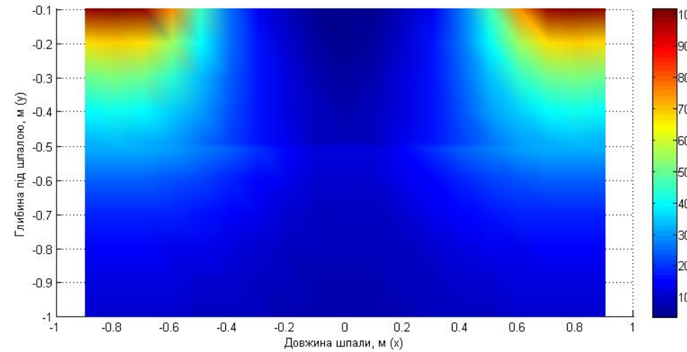
Рисунок Е.2 – Проекція розподілення напружень під шпалою № 9 ( z=0 м)
