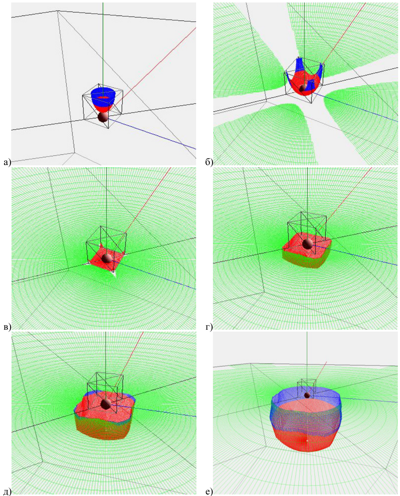
Рисунок 3.30 – Зміна обрису фронту поширення напружень при дії сили на півпростір через штамп
