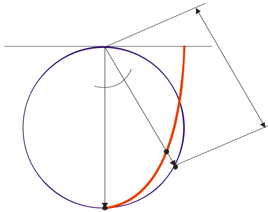
Рисунок 3.17 – Визначення функції розподілу напружень по обрису еліпсоїда
