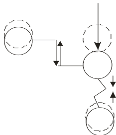
Рисунок 3.15 – Стискаючі та зсуваючі деформації речовини як переміщення елементарних часток
