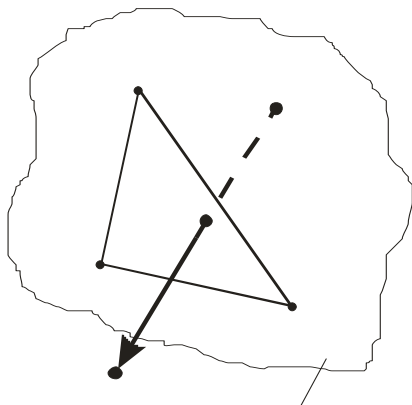
Рисунок 3.7 – Перетинання вектором площини, яка визначена рівнянням трикутника Рівняння площини будемо знаходити у вигляді
