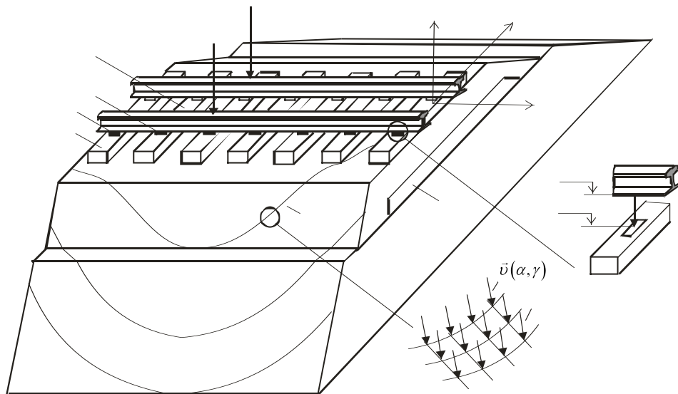
Рисунок 3.24 – Розрахункова схема для просторової моделі динамічних деформацій залізничної колії на основі теорії пружності
