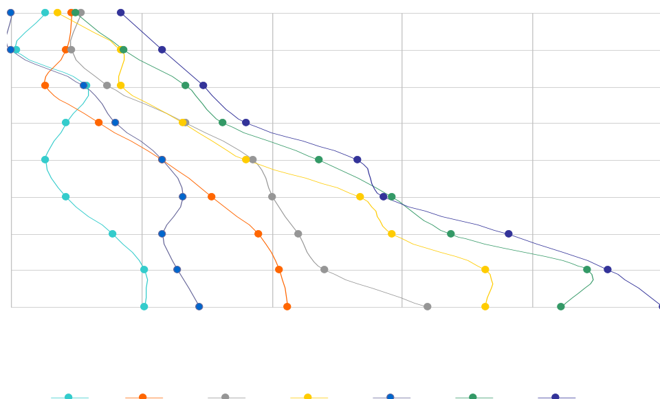
Рисунок 6.11 – Положення колеса при максимальних значеннях похідної еквівалентної роботи залізничної колії
