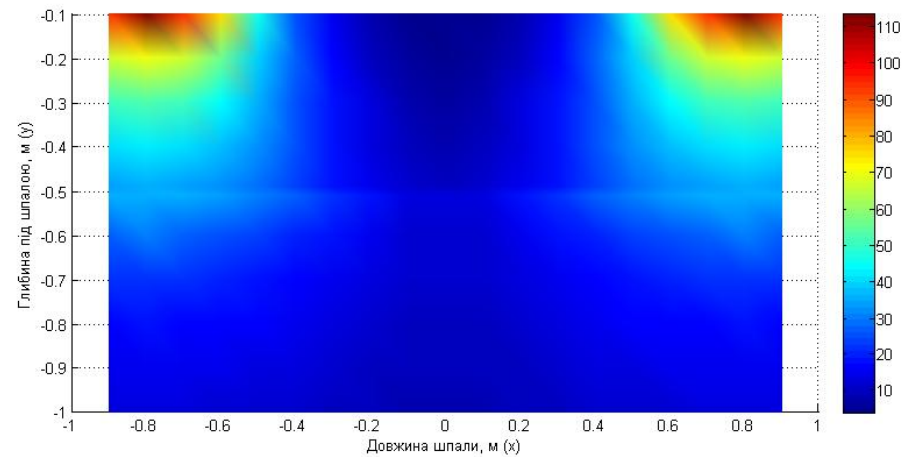
Рисунок Е.12 – Проекція розподілення напружень під шпаллюю № 10 ( z=0.54 м)
