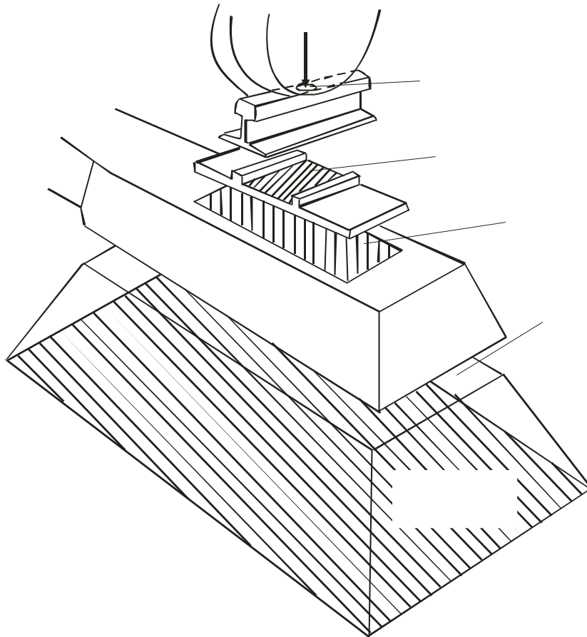
Рисунок 2.6 – Приклад розрахункової схеми для визначення напружень в елементах колії, прийнята в Угорщині [115]
