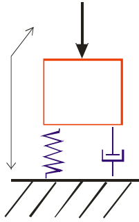
Рисунок 5.12 – Розрахункова схема роботи колії, приведеної до одного колеса
