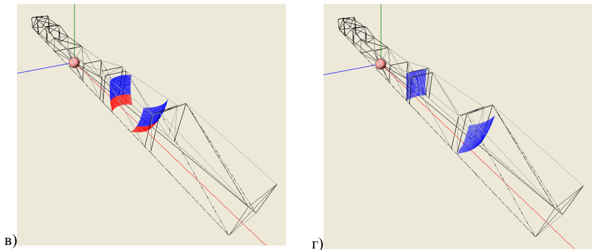
Рисунок 3.10 – Приклад обрізання простору взаємодії обрисом шпали: умовно точки поверхні, які відповідають кінцям векторів з перевагою вертикального напрямку ( 45^\circ ) показано червоним кольором, з перевагою горизонтального напрямку ( 45^\circ ) – синім.
