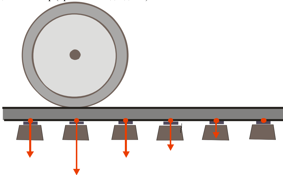
Рисунок 3.24а – Зміна сил тиску від рейки на опори, як відображення руху колеса
