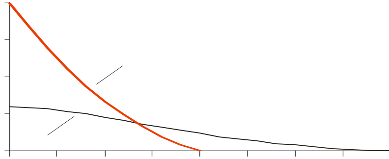
Рисунок 2.15 – Прогин рейки по довжині від точки прикладання сили: 1 – без примикання до мосту; 2 – з примиканням до мосту на відстані 1 м
