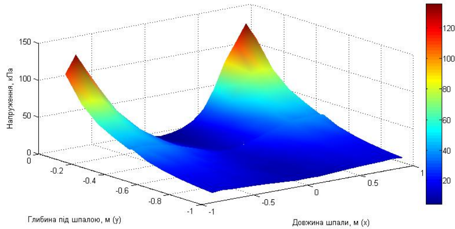
Рисунок Е.7 – Розподілення напружень під шпалою № 9 ( z=0 м)
