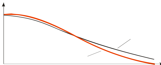
Рисунок 2.11 – Обрис розподілення навантаження по довжині рейки: 1 – для постійного значення модуля пружності ( E_0 ); 2 – для лінійного збільшення модуля пружності (від E_0 до E_1 )
