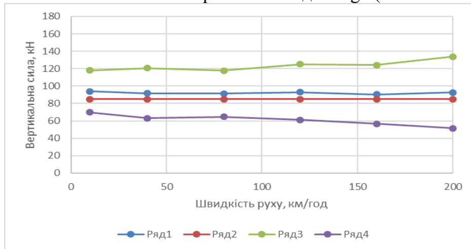
Рисунок 4.17 – Вертикальні сили за експериментальними дослідженнями для вагона пасажирського поїзда Talgo ( F_{\text{норм}} = 85 \text{ кН} )
