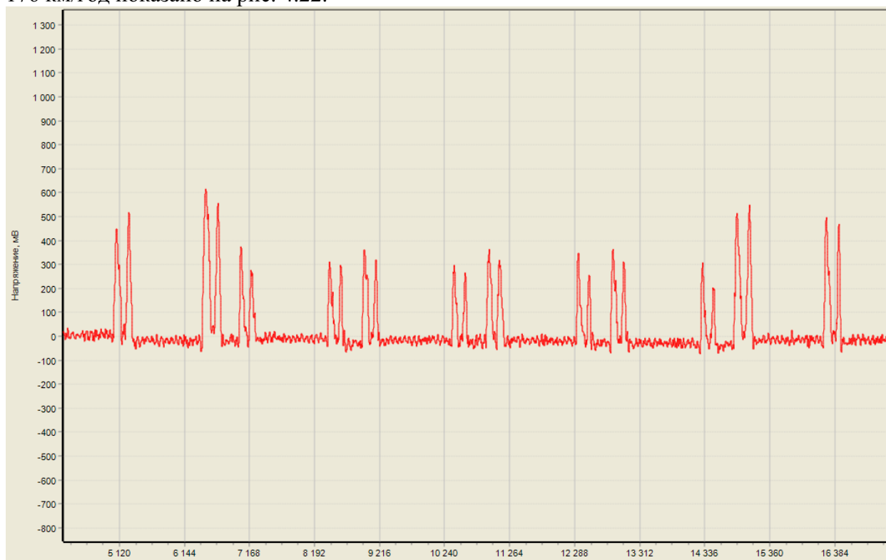
Рисунок 4.22 – Приклад запису даних з месدوزи №1 при швидкості руху 176 км/год
