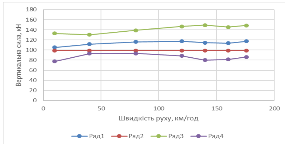
Рисунок 4.18 – Вертикальні сили за експериментальними дослідженнями для моторного вагона пасажирського поїзда Skoda ( F_{\text{норм}} = 99 \text{ кН} )
