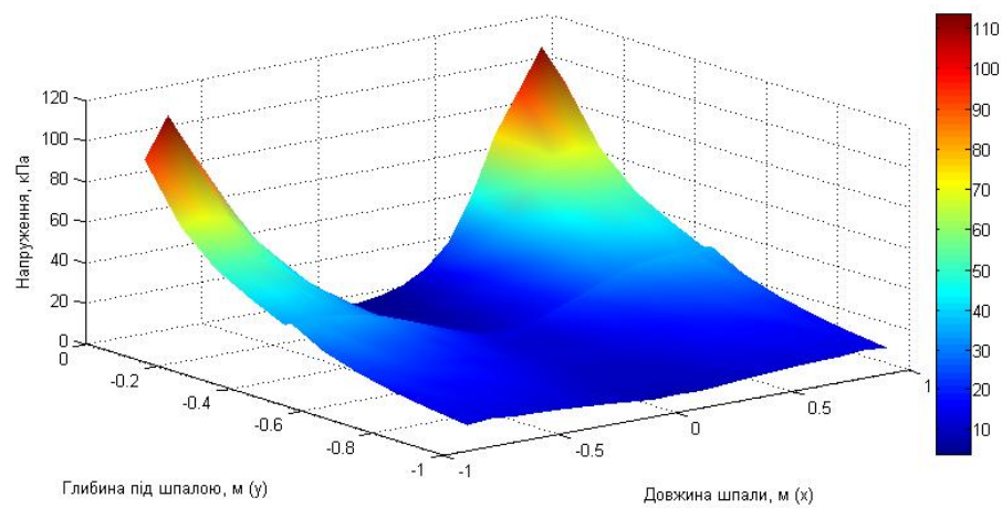
Рисунок Е.11 – Розподілення напружень під шпаллюю № 10 ( z=0.54 м)
