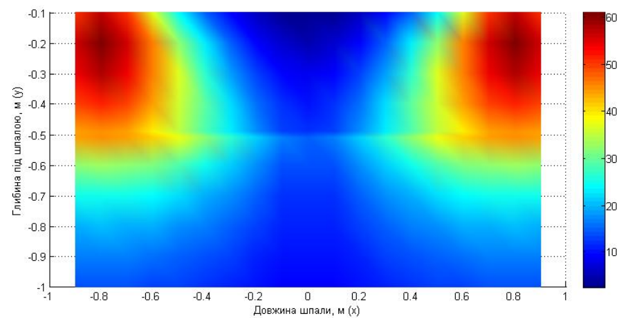
Рисунок Е.10 – Проекція розподілення напружень між шпалами № 9 і 10 ( z=0.27 м)
