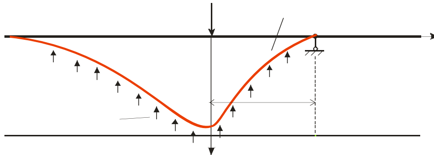
Рисунок 2.14 – Розрахункова схема прогину балки на ділянці підходу до моста
