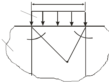
Рисунок 2.1 – Схема дії рівномірно розподіленого навантаження, яке прикладене на поверхні напівпростору
