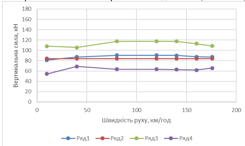
Рисунок 4.18 – Вертикальні сили за експериментальними дослідженнями для моторного вагона пасажирського поїзда Skoda ( F_{\text{норм}} = 99 \text{ кН} )
