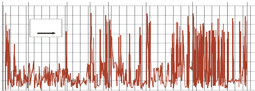
Рисунок 2.21 – Зміна механічної роботи сили тяги локомотива при русі пасажирського поїзда за напрямком Київ - Львів
