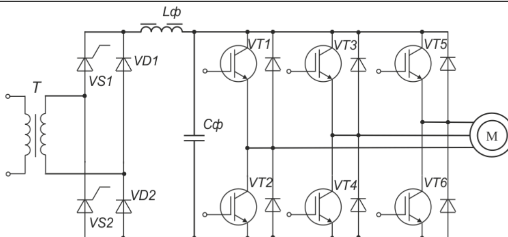
Рис. 2. Предлагаемая схема преобразователя асинхронных приводов вспомогательных механизмов
