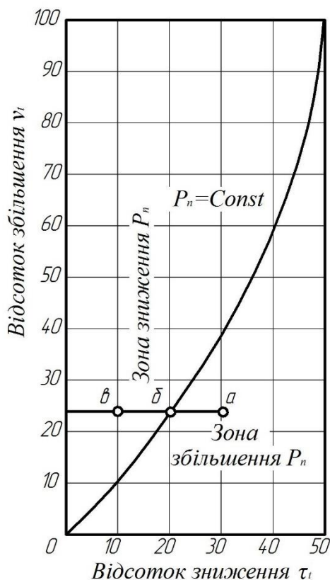
Рис. 2.3. Вплив на корисну роботу локомотива P_k процентних змін швидкості руху V_m та питомого простоя на станціях \tau_t .
