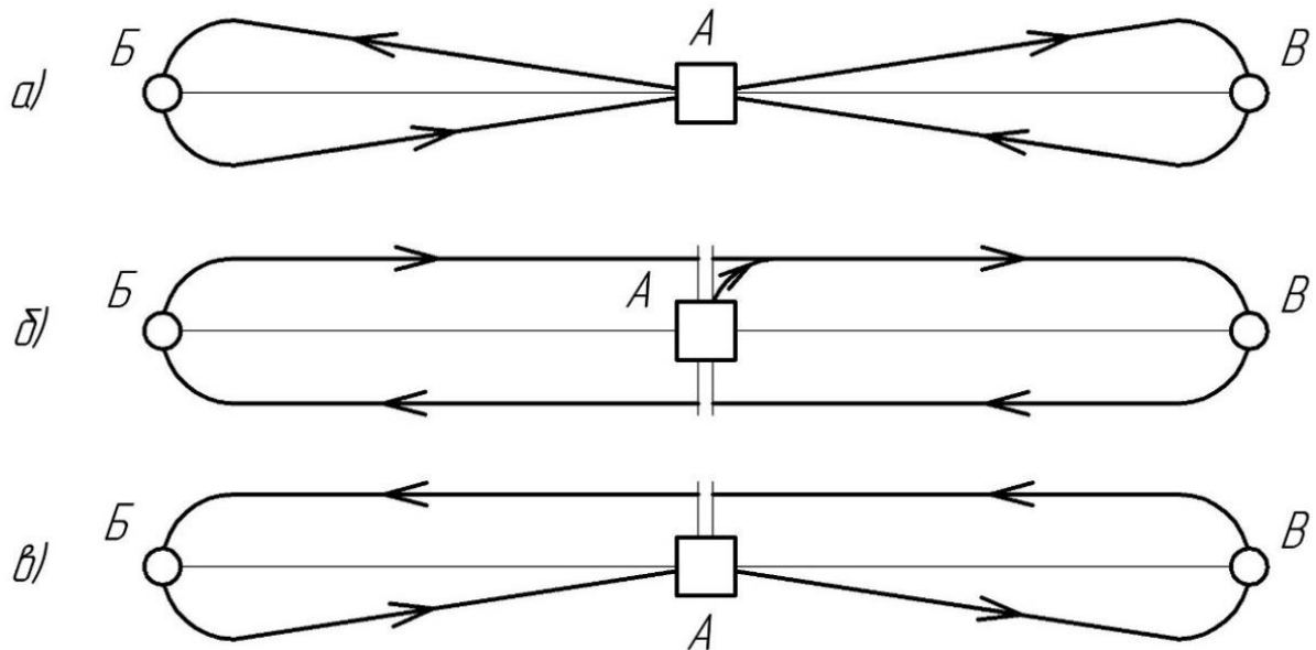
Рис. 1.1. Способи обслуговування, поїздів локомотивами:
