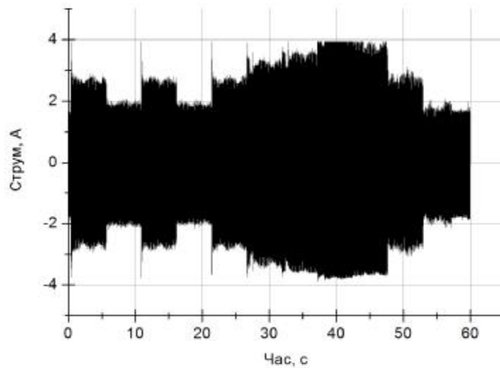
Рис.1. Узагальнена осцилограма зміни вхідного струму за частоти модуляції 1 кГц
