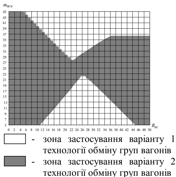
Рис. 4. Зони раціонального застосування варіантів технології обміну груп вагонів у залежності від впливаючих факторів при наявності зміни поїзного локомотива
