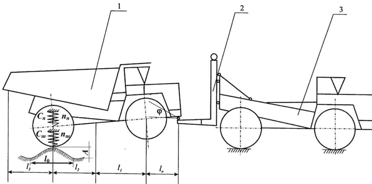
Рисунок 2 – Схема буксирування захватом спереду
