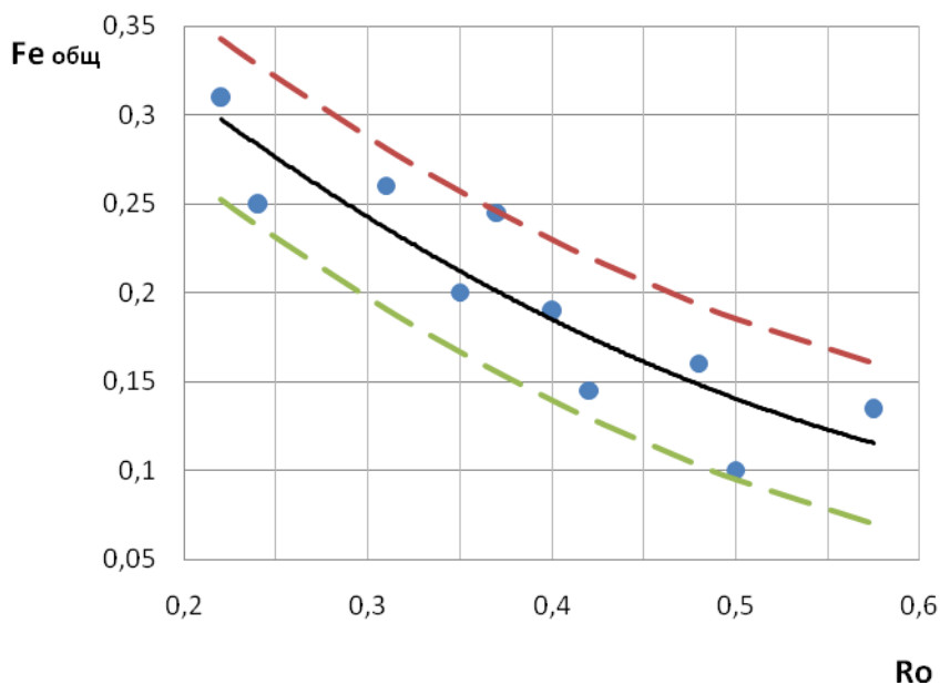
Рис. 2. Зависимость содержания железа общего в шлаке от его отражательной способности
