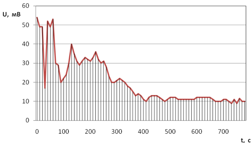
Рис. 1. Изменение величины отраженного сигнала радара по ходу продувки
