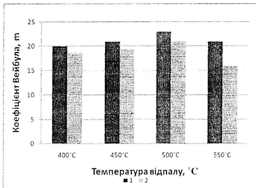
Рис. 1. Вплив технологічної і термічної обробки на коефіцієнт гомогенності Вейбула ( m ) дослідженої сталі: 1 — головка зразка; 2 — зона рівномірного видовження
