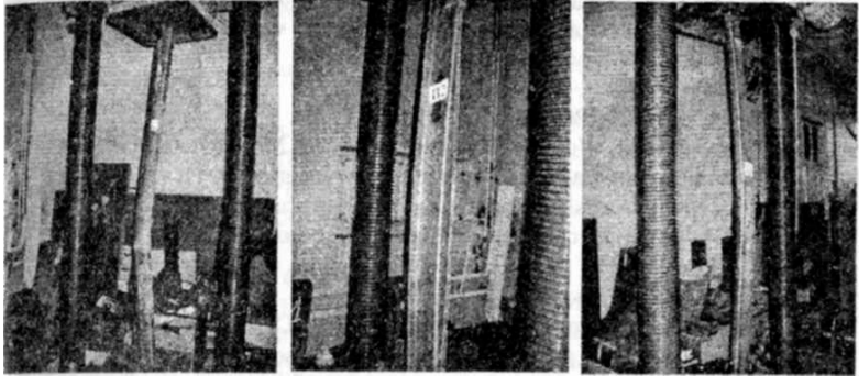
Рис. 4. Втрата стійкості стержнів під навантаженням
