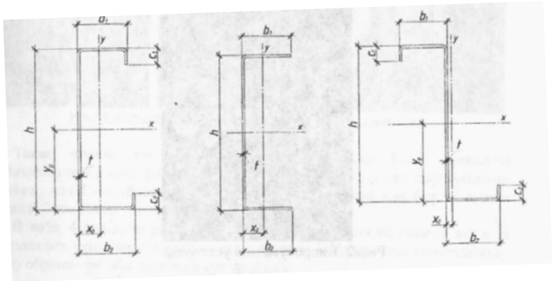
Рис. 1. Поперечний переріз стержнів, що досліджувалися
