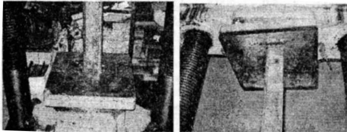
Рис. 3. Закріплення стержня
