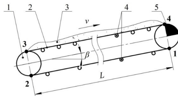
Рисунок 1 – Схема конвеєра: 1 – натяжний барабан; 2 – стрічка; 3 – транспортований вантаж; 4 – ролик; 5 – приводний барабан
