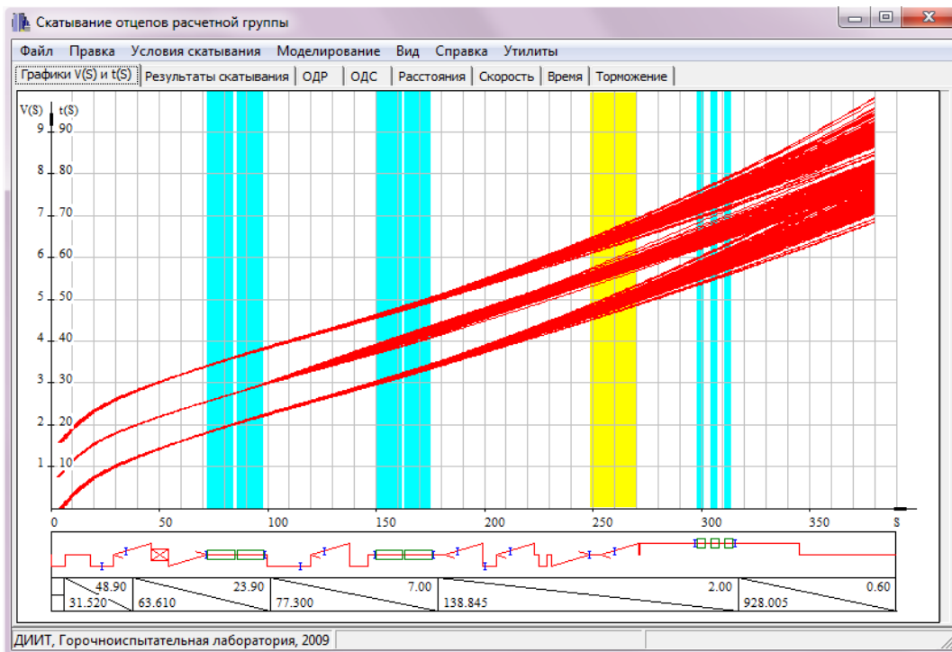
Fig. 1. Main window of the software, simulating cuts rolling from the gravity hump Рис. 1. Главное окно программы, моделирующей скатывание отцепов с сортировочной горки
