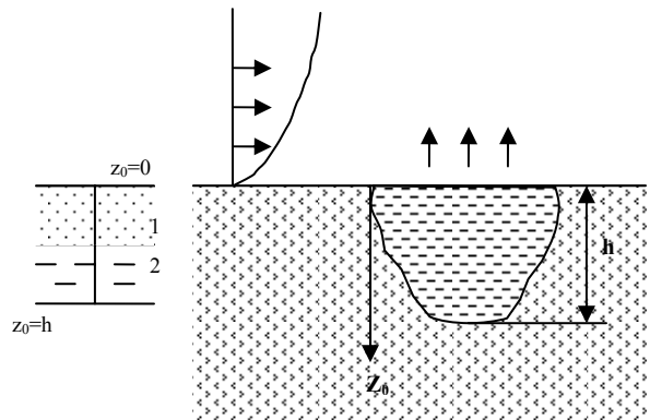
Рис. 2. Схема зоны загрязнения грунта
