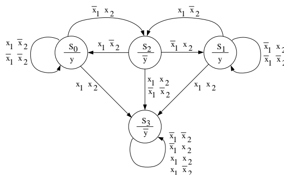
Рис. 6.Орієнтований граф дискретного автомату що описує роботу стрілочного переводу
